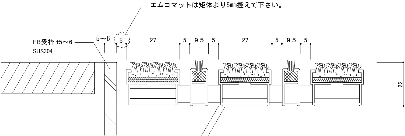
522/RB タイプ 断面詳細図S=1:1
