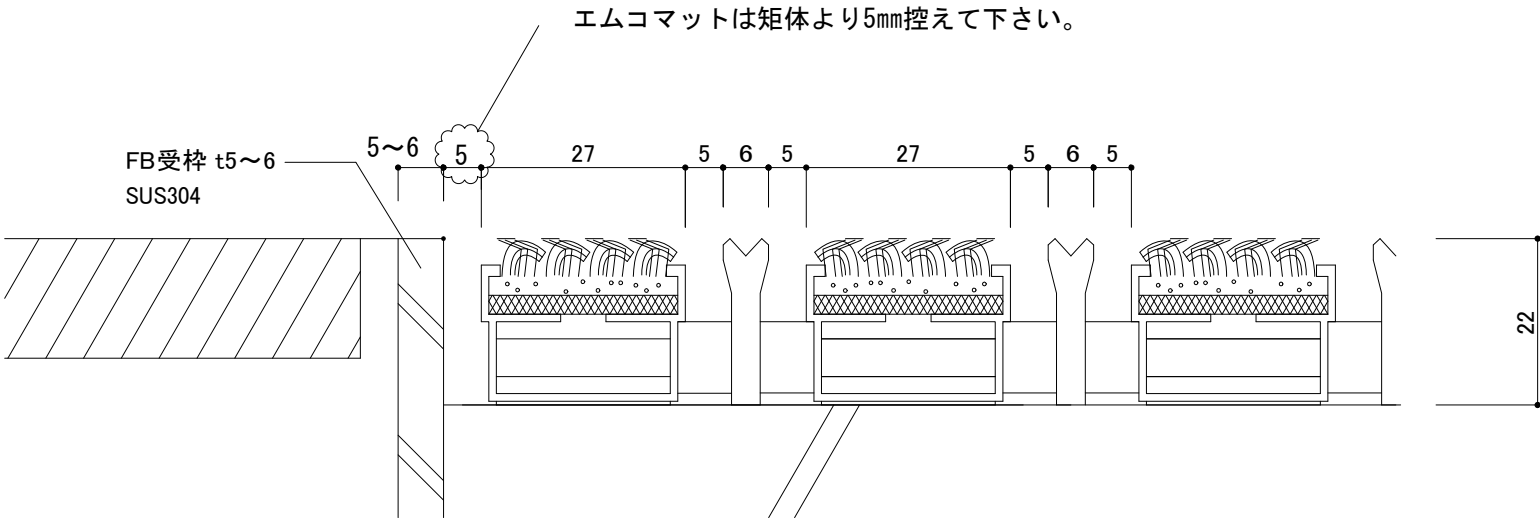
522/RK タイプ 断面詳細図S=1:1
