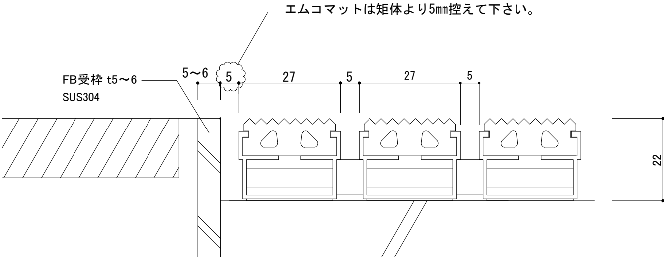
522/G タイプ 断面詳細図S=1:1
