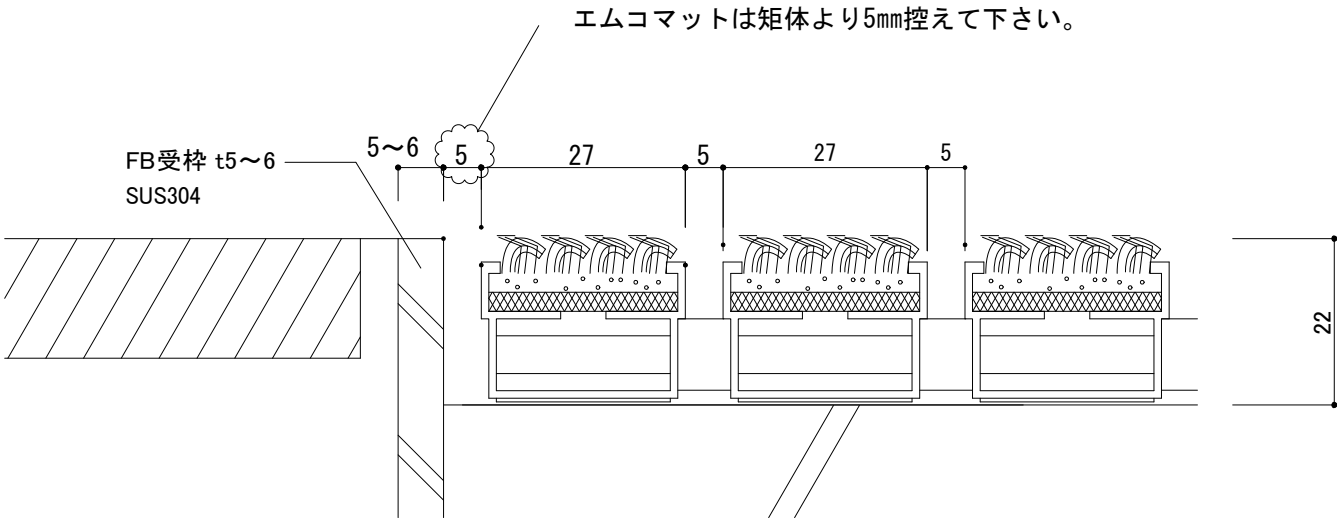
522/R タイプ 断面詳細図S=1:1
