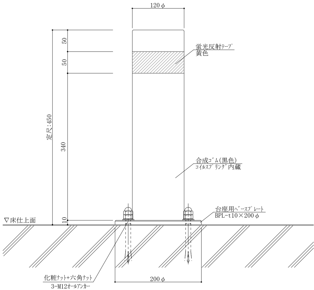
GP-450Y(合成ゴム・コイルスプリング内蔵) 詳細図
