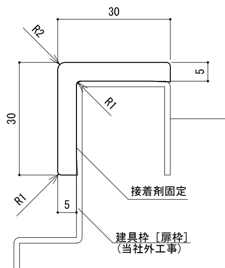
コーナーガード : AKC-30
