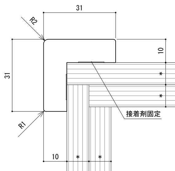
コーナーガード : AKC-31B
