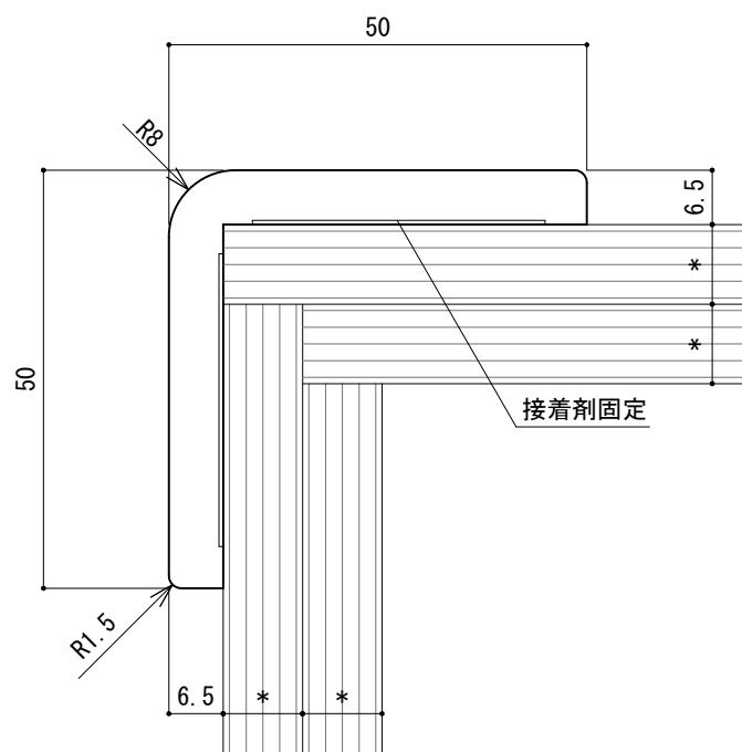
コーナーガード : AKC-50A
