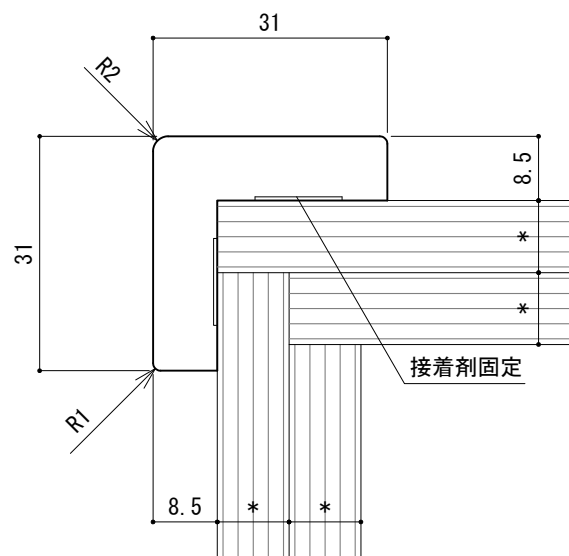
コーナーガード : AKC-31A
