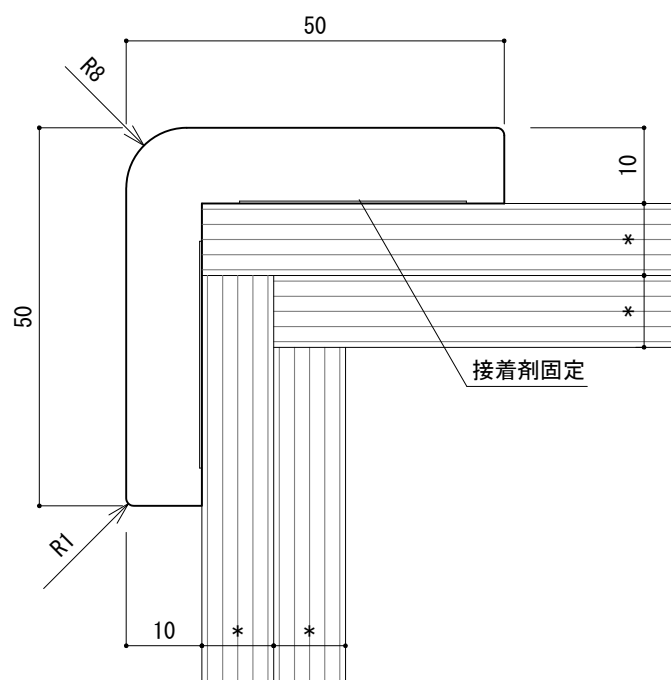
コーナーガード : AKC-50B
