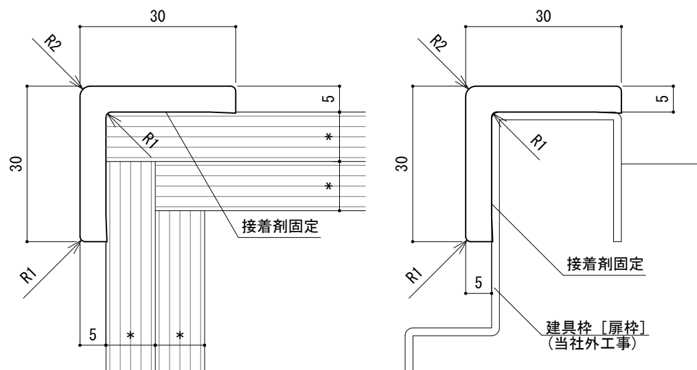
コーナーガード : AKC-30
