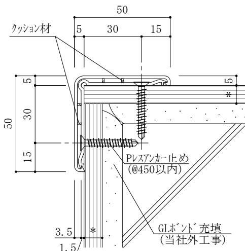
RC下地 PB*(GL工法)
