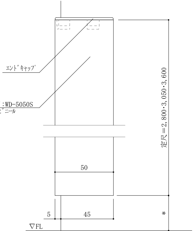
立面図
