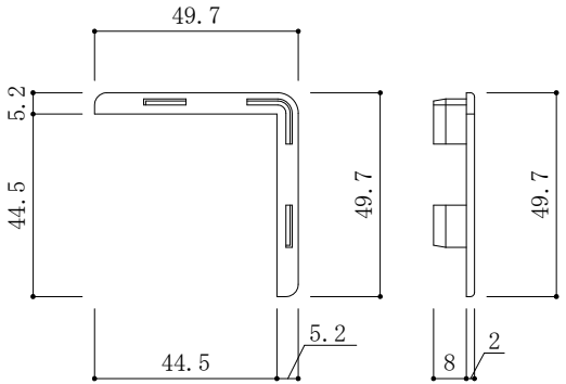
WD-5050S用エンドキャップ (材質：硬質塩化ビニール・抗菌剤配合)
