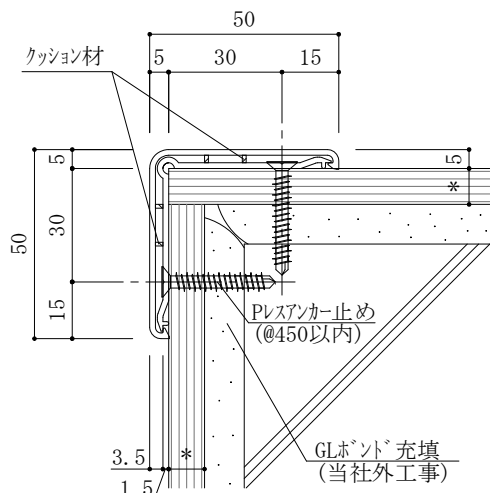
RC下地 PB*(GL工法)
