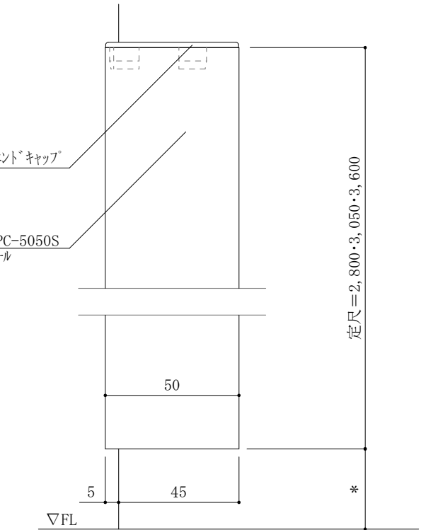
立面図
