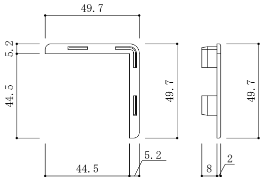
APC-5050S用エンドキャップ (材質：硬質塩化ビニール・抗菌剤配合)
