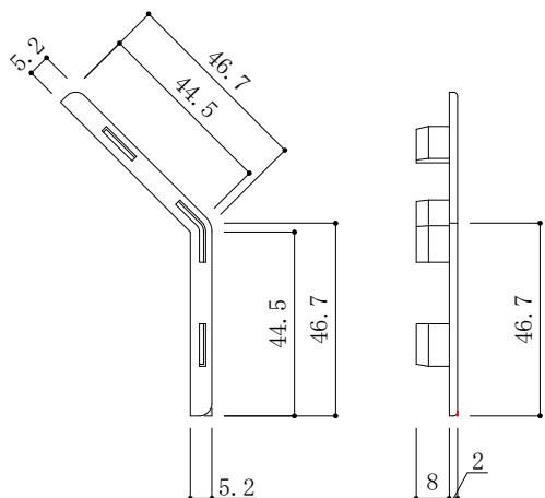
APC-5050S用エンドキャップ (135° 用) (材質：硬質塩化ビニール・抗菌剤配合)
