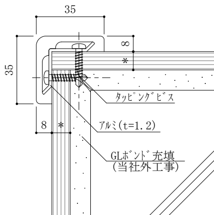
RC下地 PB* (GL工法)
