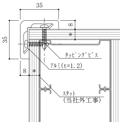
LGS下地 PB*
