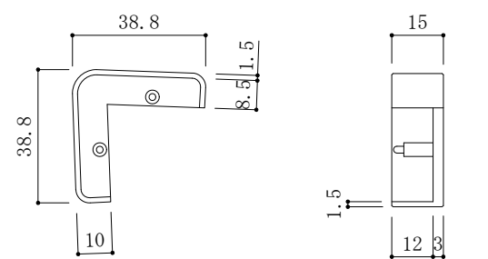
APC-3535V用 エントキャップ (材質:塩化ビニール)
