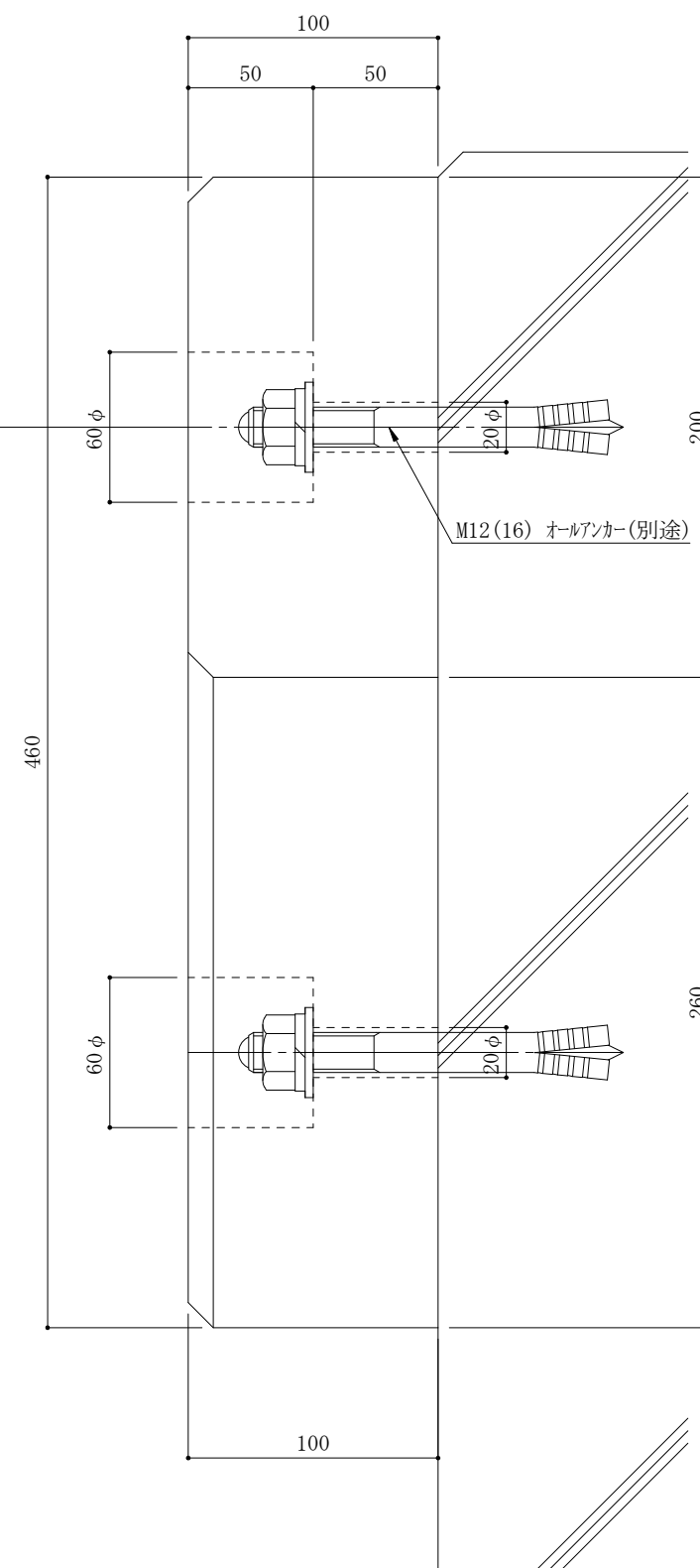
ACL-1246 断面図
