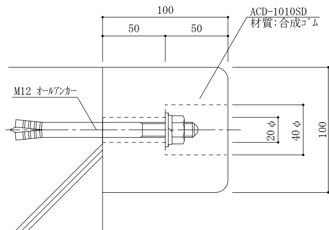
ACD-1010SD 断面図
