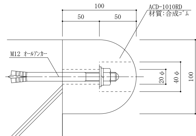
ACD-1010RD 断面図
