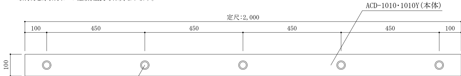
ACD-1010Y(黄色ライン入り) 詳細図
