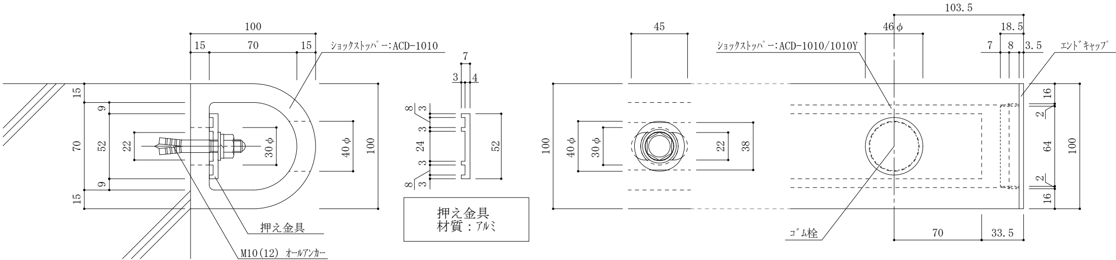
ACD-1010 詳細図
