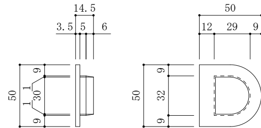
エンドキャップ 詳細図
