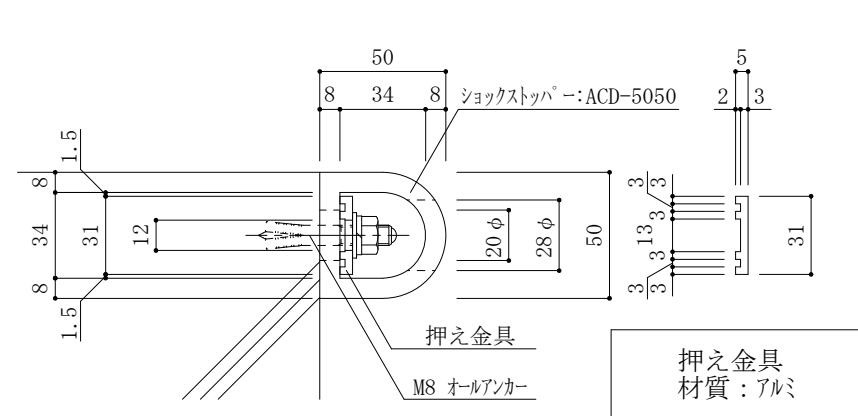
ACD-5050 詳細図
