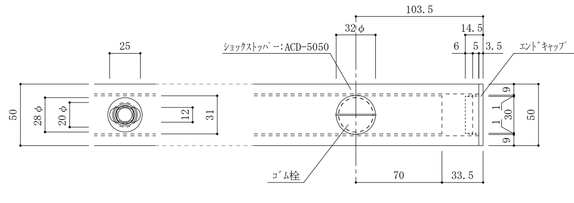
各部材展開(正面)図
