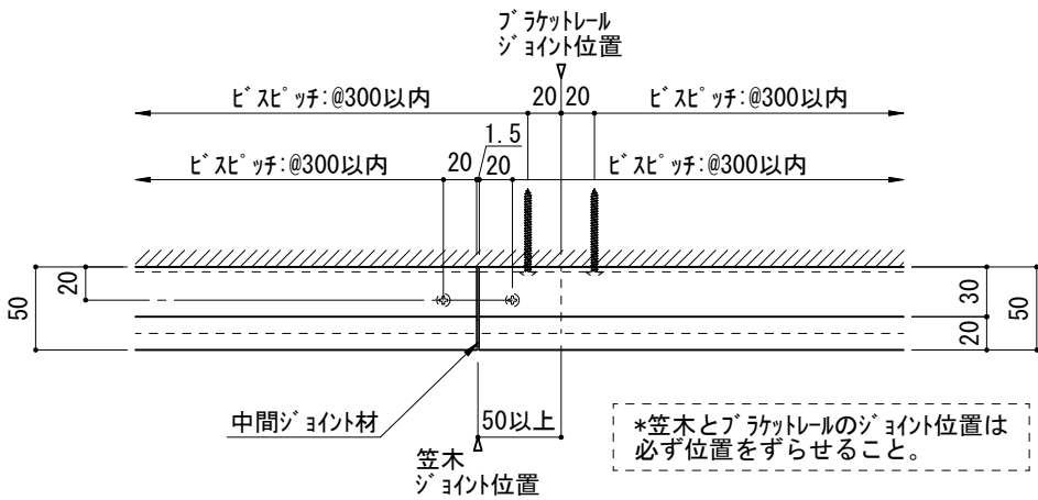
エライン：AL-102 中間ジョイント部 平面納まり図
