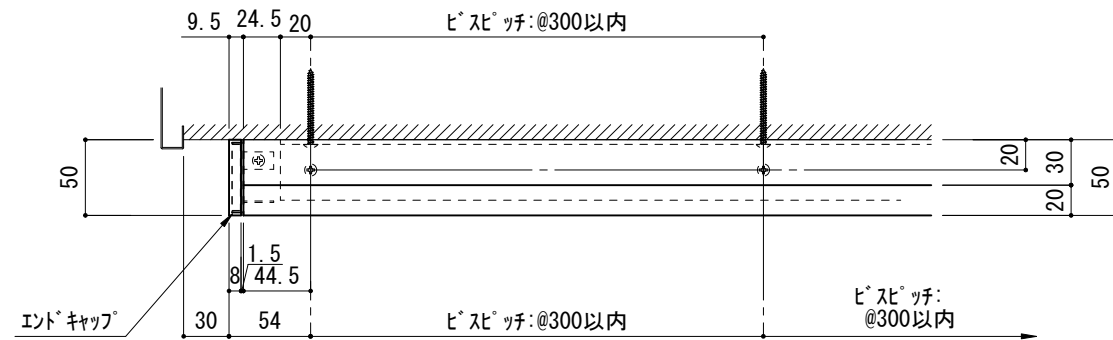
エライン：AL-102 端部 平面納まり図
