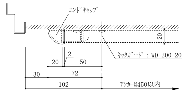
端部平面詳細図
