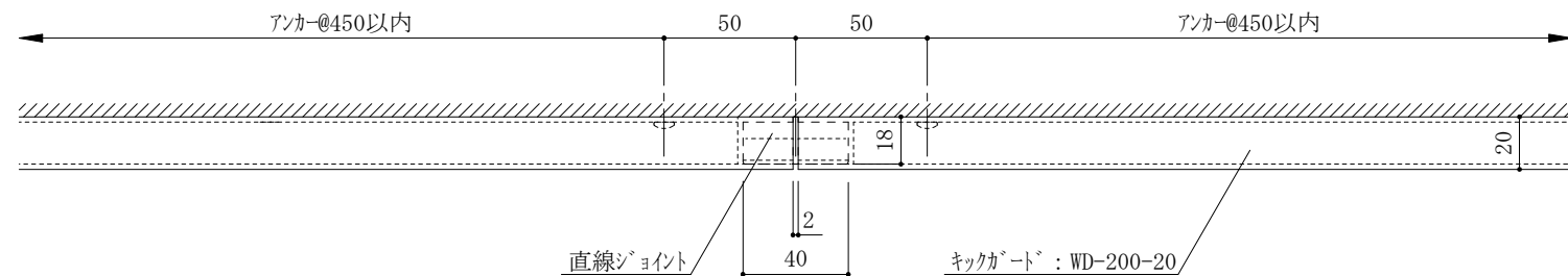
直線ジョイント部平面詳細図
