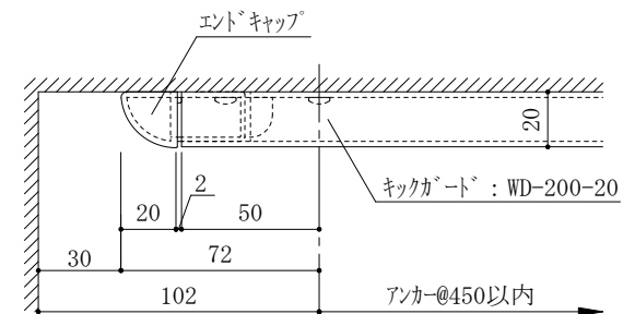
端部平面詳細図
