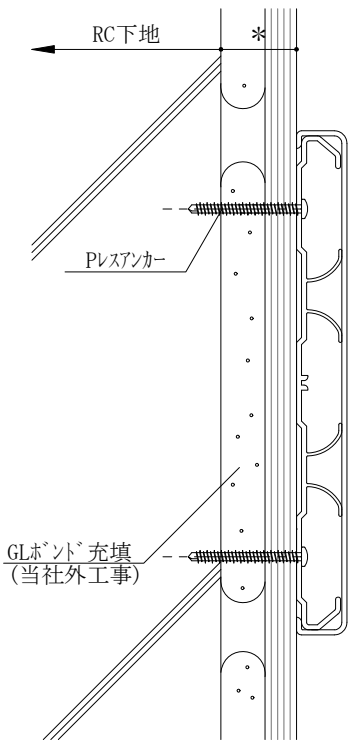
RC下地 PB*(GL工法)
