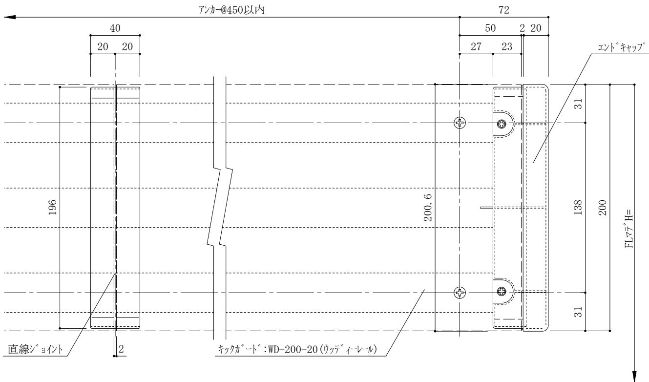
各部材展開(正面)図
