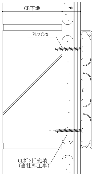
CB下地 PB*(GL工法)
