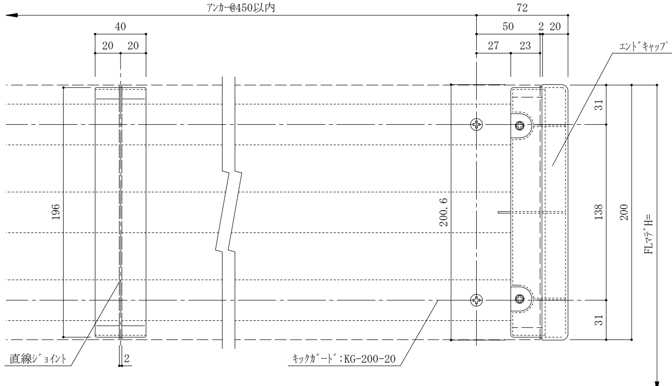
各部材展開(正面)図
