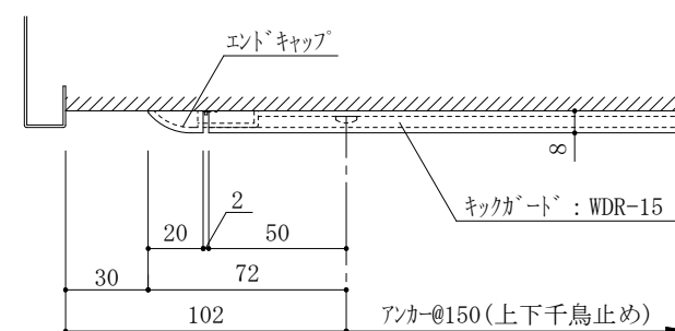
端部平面詳細図
