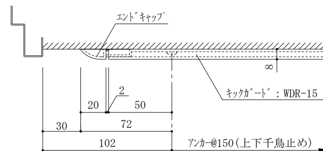
端部平面詳細図
