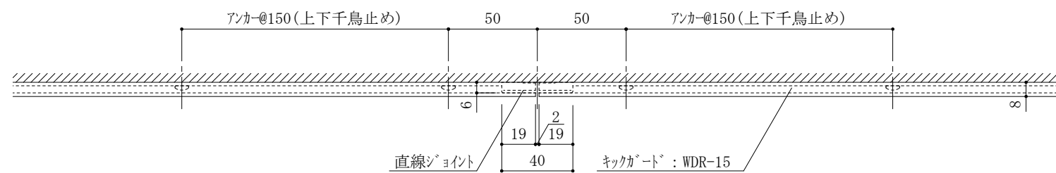
直線ジョイント部平面詳細図
