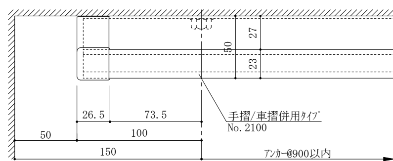
端部平面詳細図
