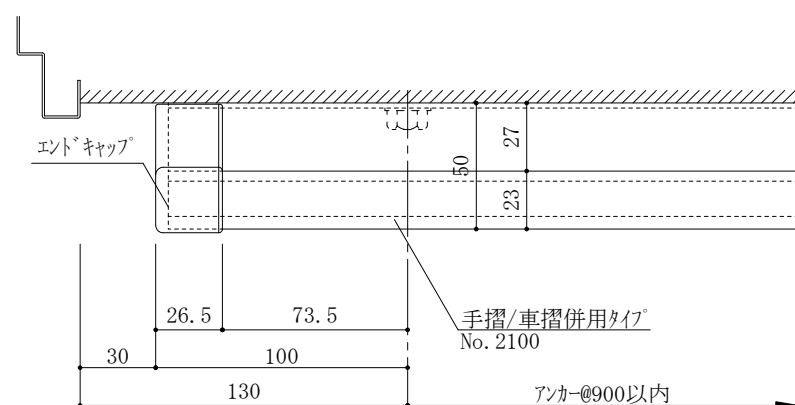
端部平面詳細図
