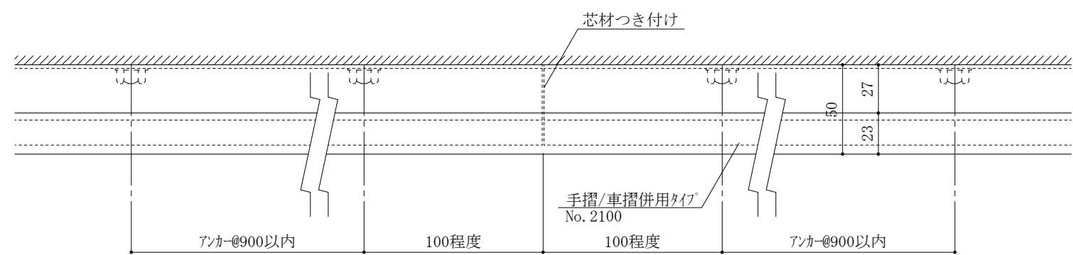
直線ジョイント部(芯材)平面詳細図
