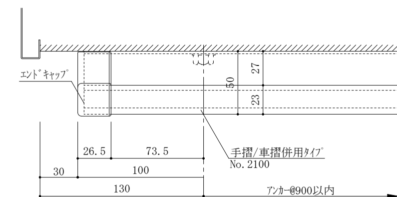
端部平面詳細図
