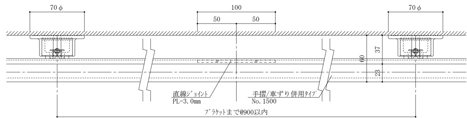
直線ジョイント部平面詳細図
