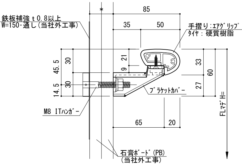
LGS壁(鉄板補強)+石膏ボード* AG-105・ブラケットB:取付断面施工例
