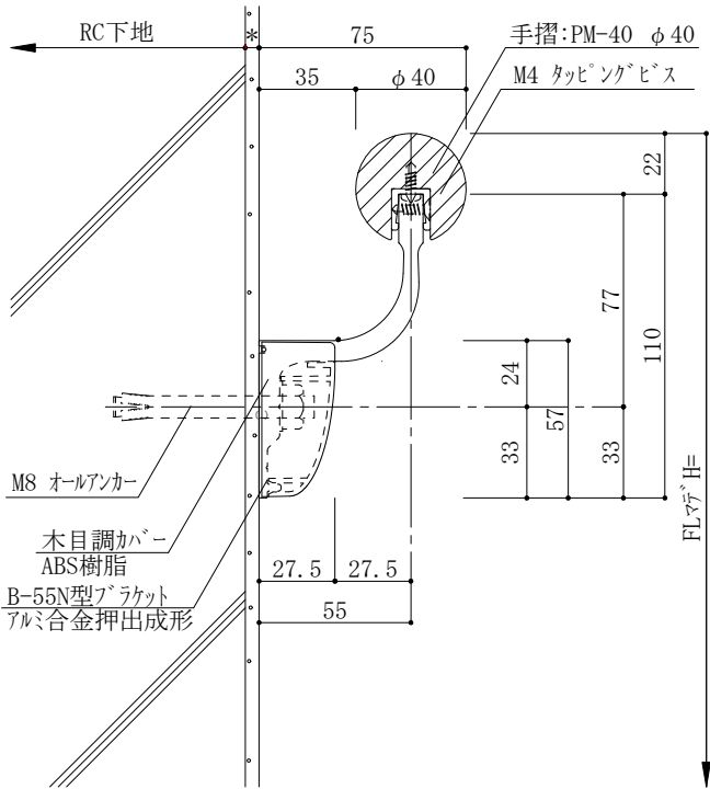
RC下地 取付断面詳細図
