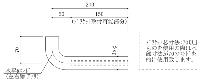
端部平面詳細図
