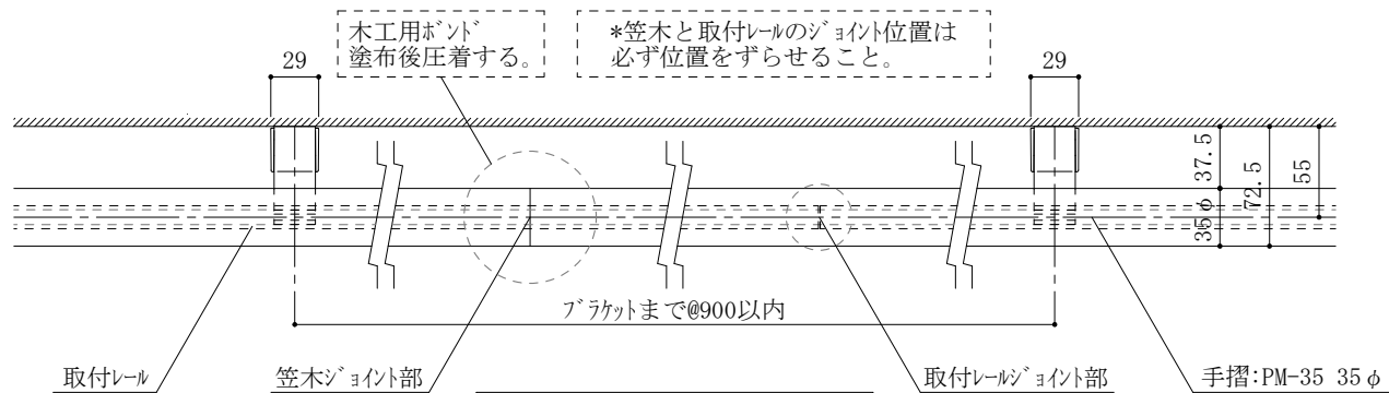
直線ジョイント部平面詳細図
