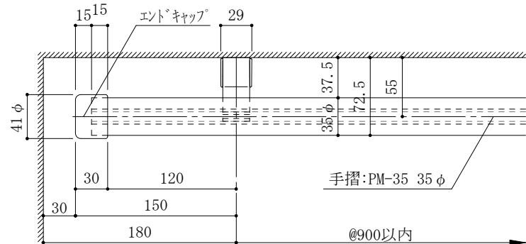
端部平面詳細図
