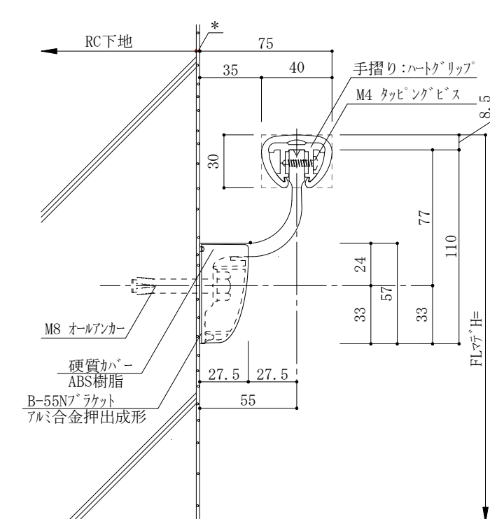
RC下地 取付断面
