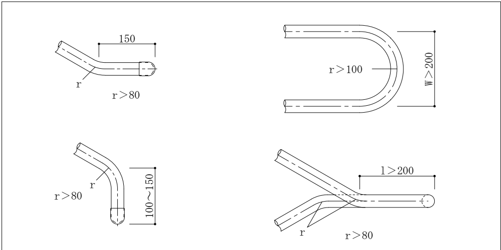
曲げ加工例
