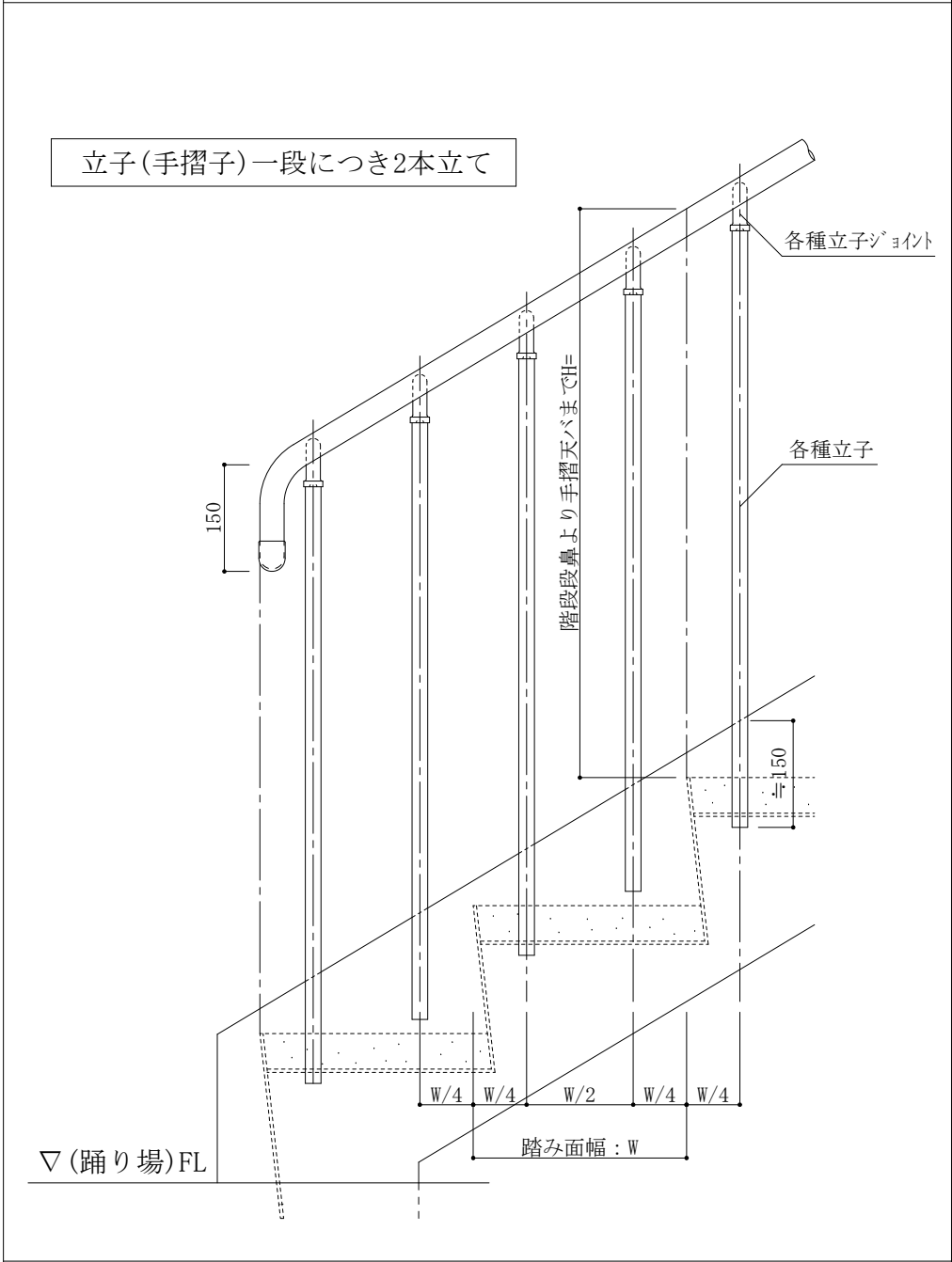
階段立子付手摺取付例
