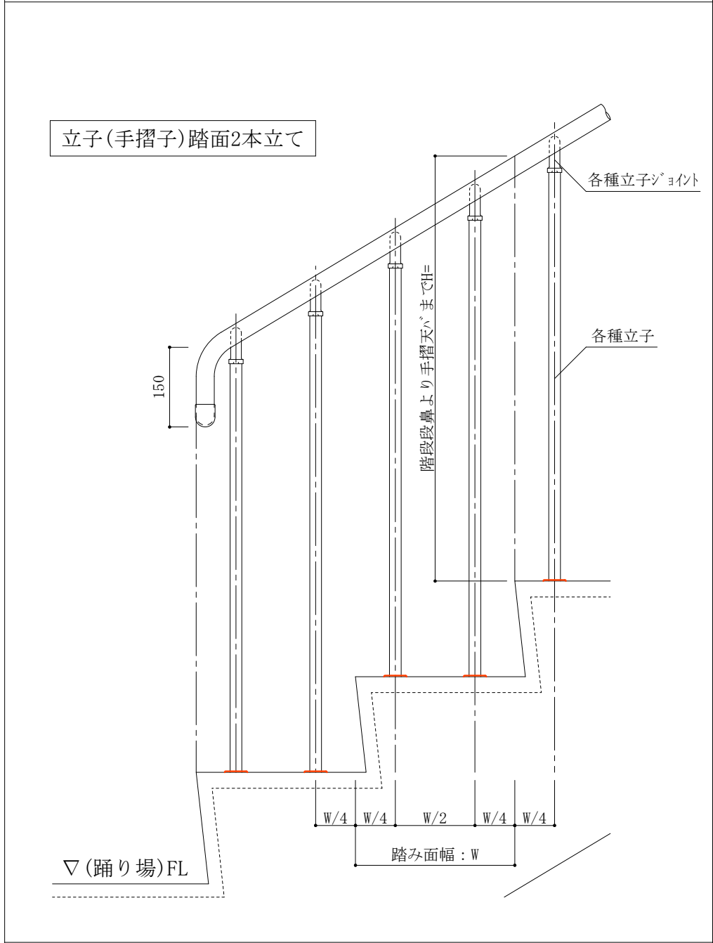
階段立子付手摺取付例
