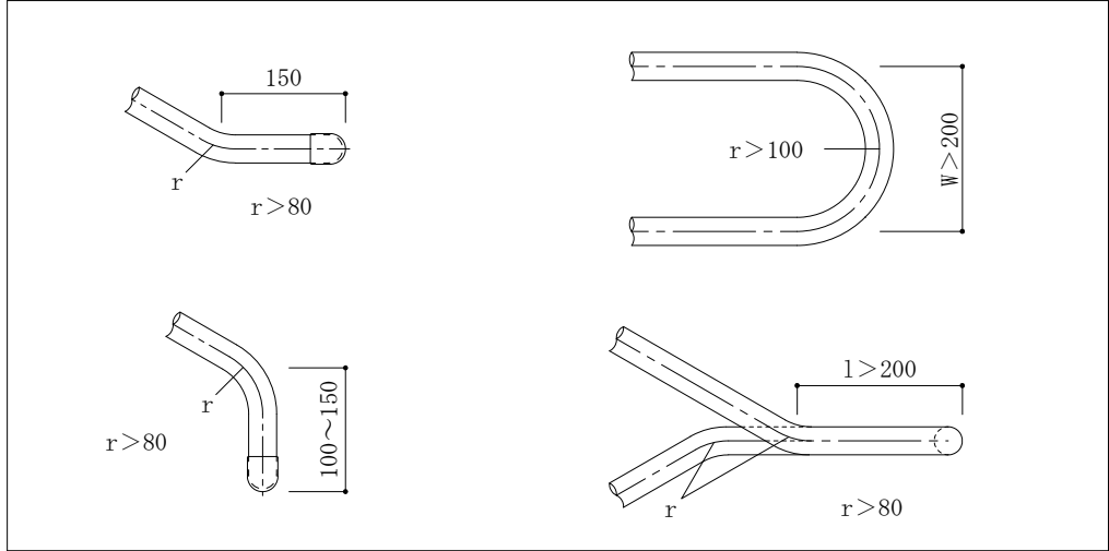
曲げ加工例
