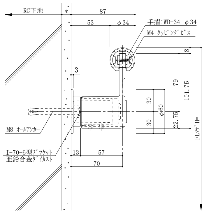
ブラケット:I-70-6型(亜鉛合金ダイカスト製品)
