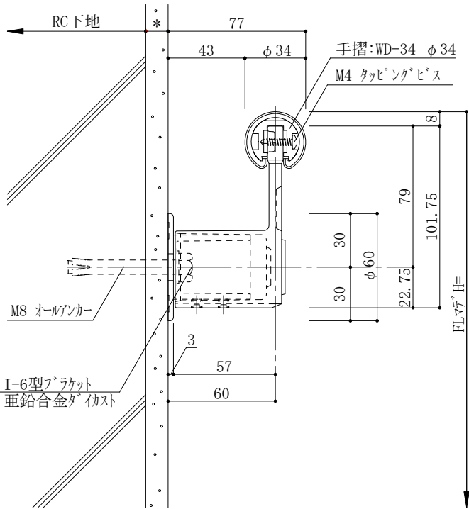
ブラケット展開(正面)図
