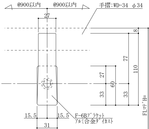
ブラケット展開(正面)図
