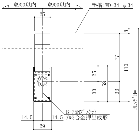
ブラケット展開(正面)図
