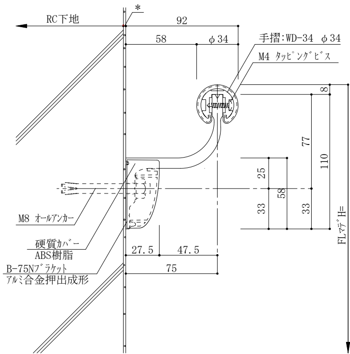
RC下地 取付断面図
