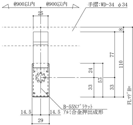
ブラケット展開(正面)図
