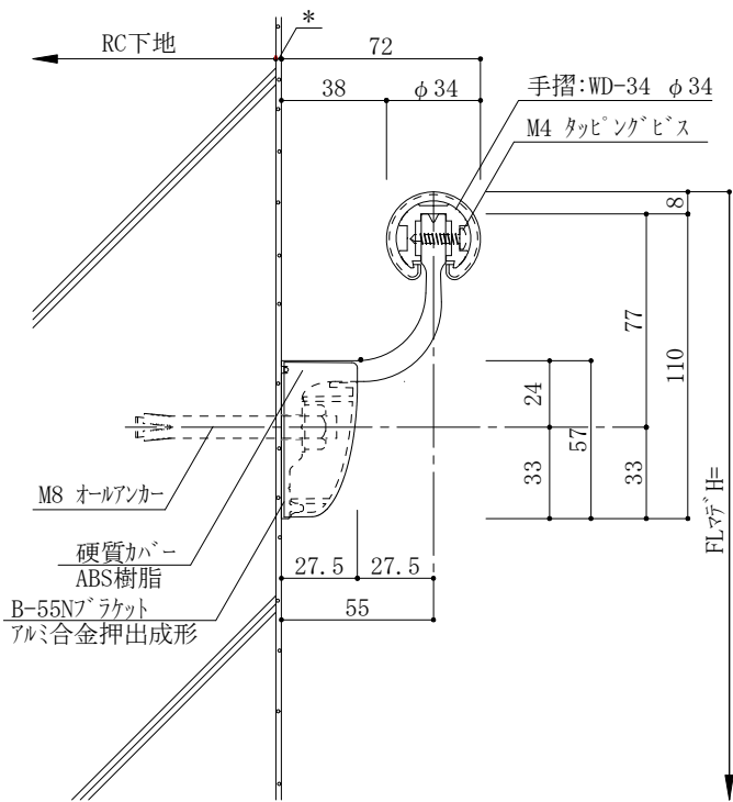
RC下地 取付断面図
