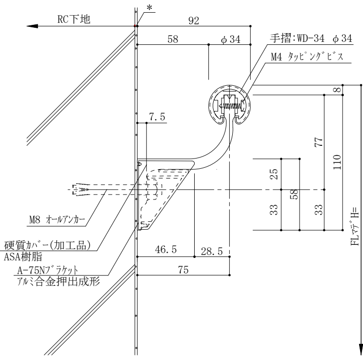
RC下地 取付断面図
